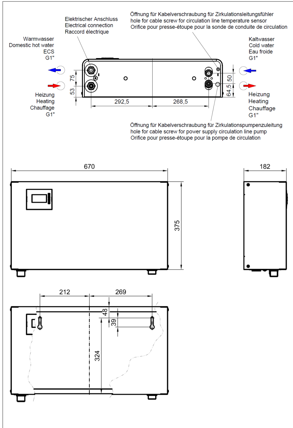
Figure 5 : Cotes de raccordement en mm, (vue de dessous)
