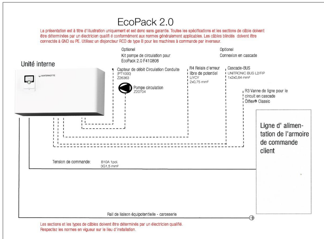
Figure 6 : Liste des câbles – EcoPack 2.0
