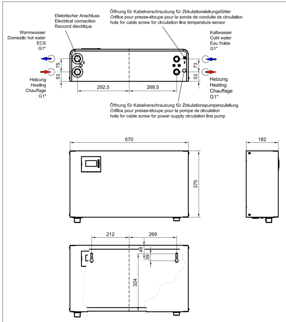
Abbildung 4: Anschlussmaße in mm
