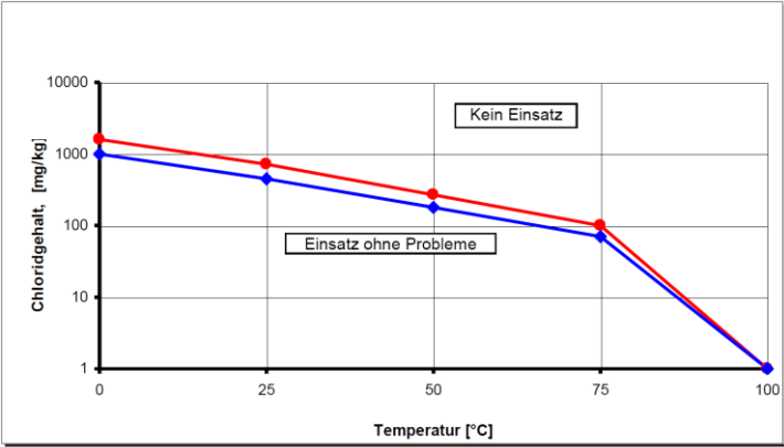
Abbildung 7: Zulässiger Chloridgehalt in Abhängigkeit der Temperatur
