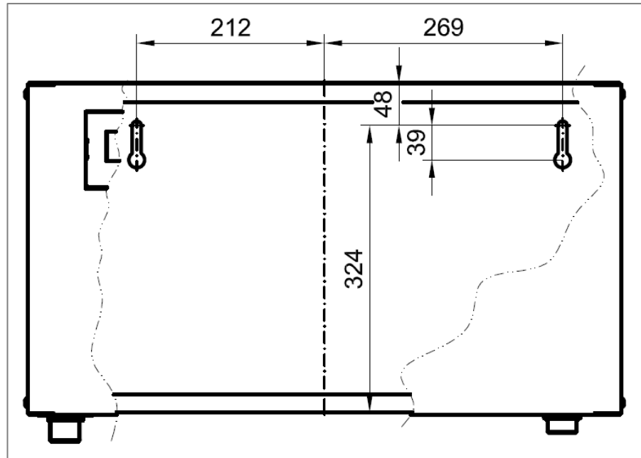
Figure 3 : Schéma de perçage pour la fixation au mur du chauffe-eau instantané
