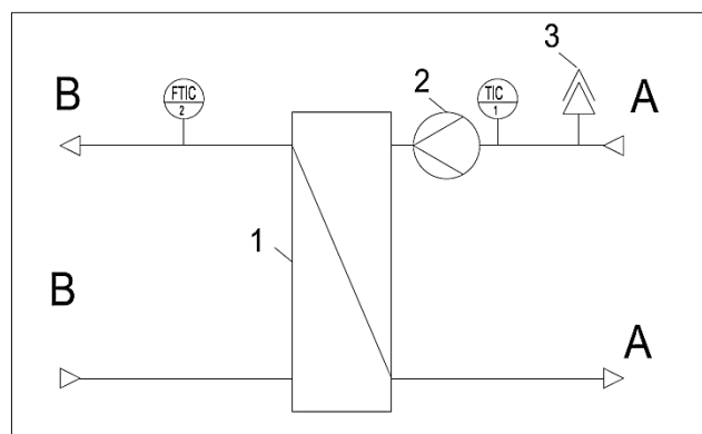
Abbildung 1: Elektronischer Kompakt-Trinkwassererwärmer
