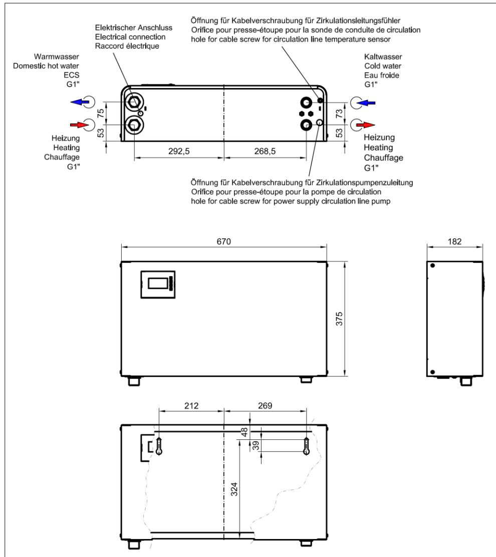
Figure 4 : Cotes de raccordement en mm, (vue de dessous)
