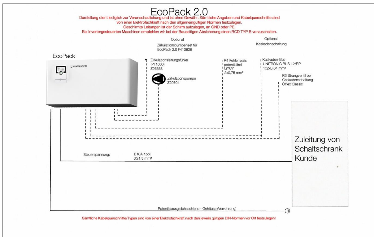
Abbildung 6: Kabelzugliste EcoPack 2.0
