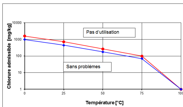
Figure 7 : Résistance à la corrosion (des plaques inox) au chlorure en fonction de la température
