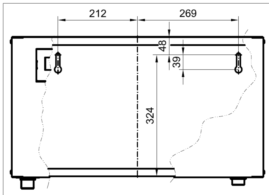
Abbildung 3: Bohrbild Kompakt-Trinkwassererwärmer
