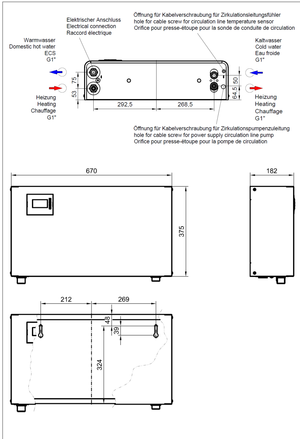
Abbildung 5: Anschlussmaße in mm
